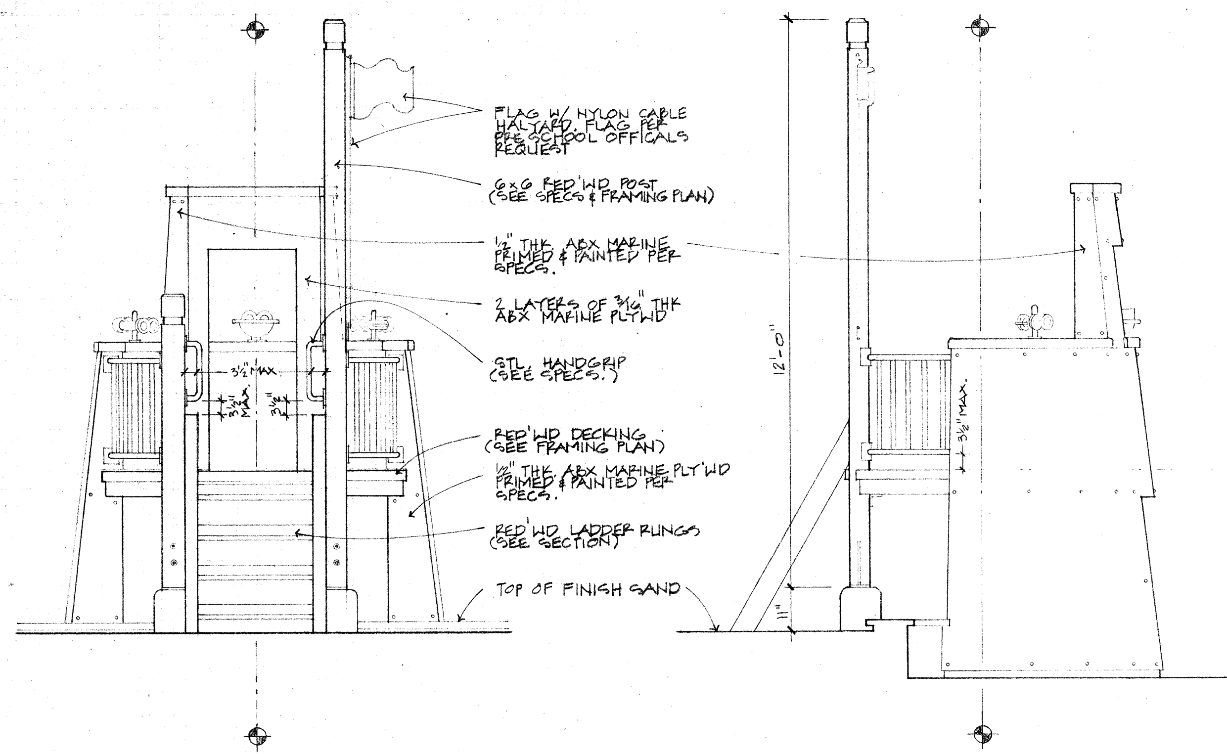
Elevation I
